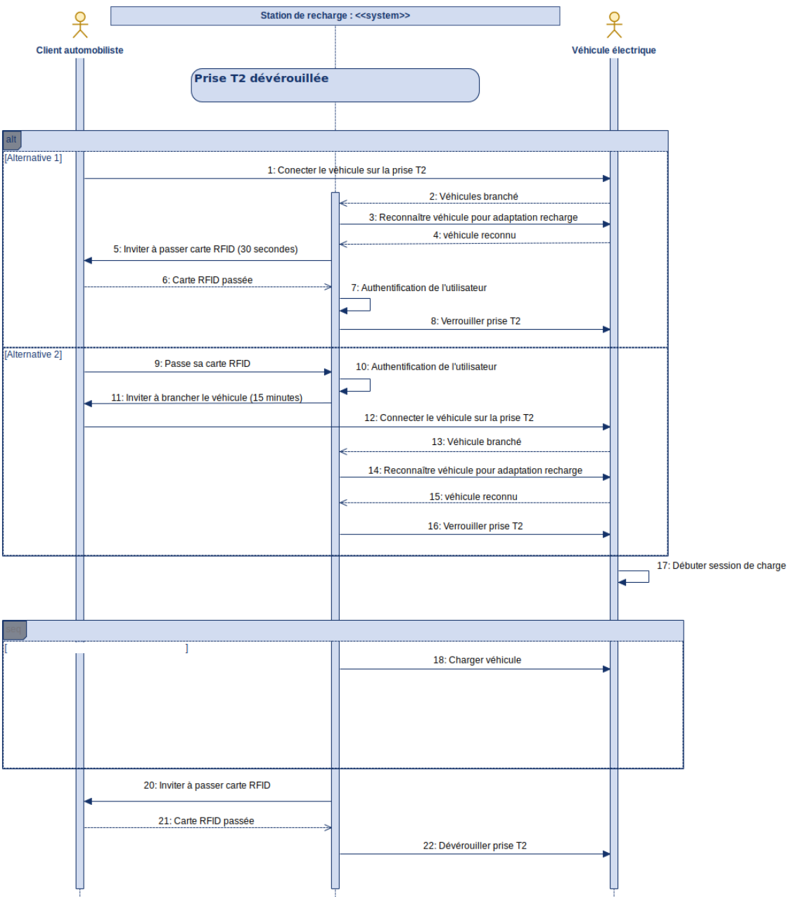
Figure 5: Diagramme d'activité système
