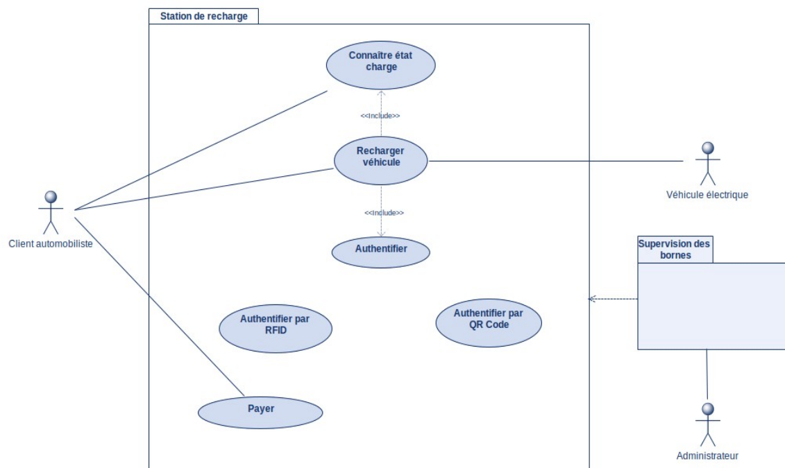
Figure 4: diagramme de cas d'utilisation – Station de recharge
